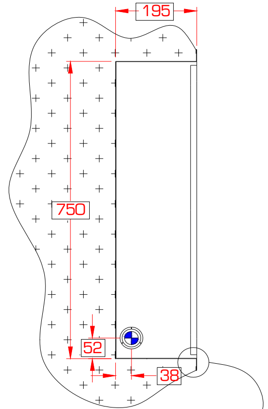
DETALLE A
